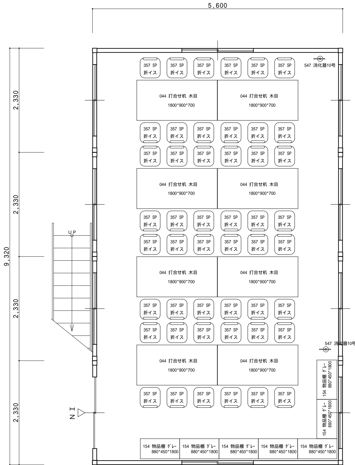
1 F 平面図
